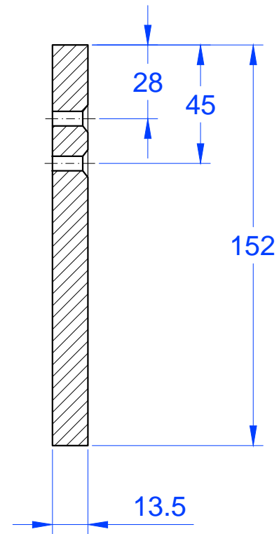
Schnitt A-A
